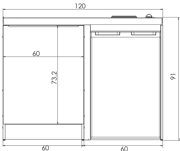
Vue face
